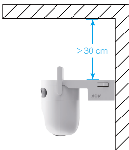
圖 2 壁掛式安裝
