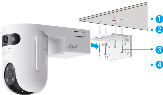
圖 1 天花板安裝
